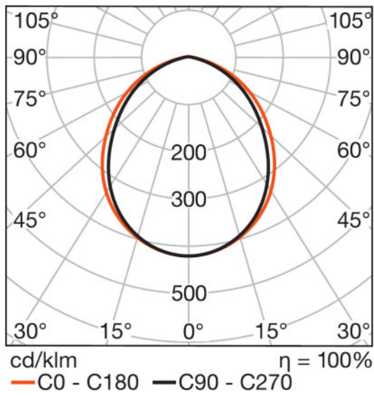
Courbe photometrique, polaire
