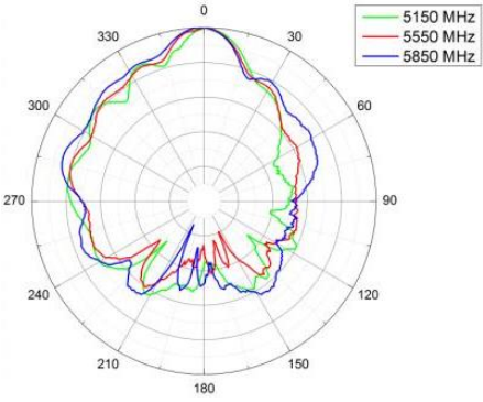
Port2: E-Plane
