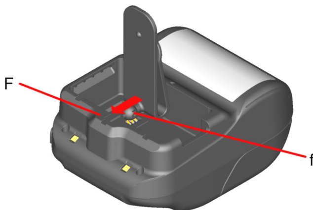
Abbildung 15-1 Anbringung des Gürtelclips (1)
