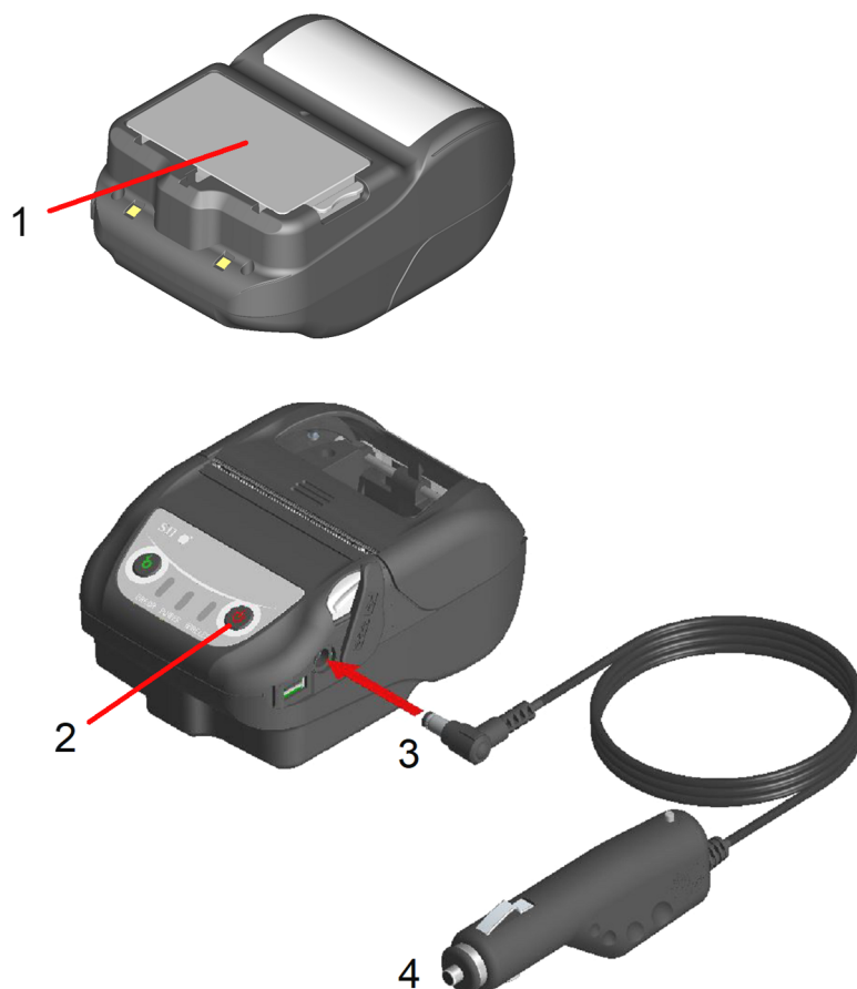
Abbildung 18-2 Aufladen im eingeschalteten Lademodus mit dem Kfz-Ladegerät
