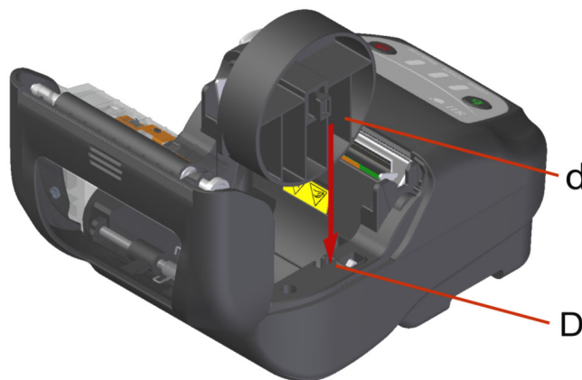
Abbildung 14-1 Anbringen der Trennwand
