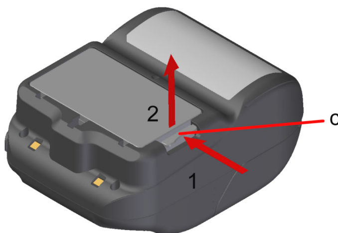
Abbildung 8-1 Entnehmen des Akkupakets
