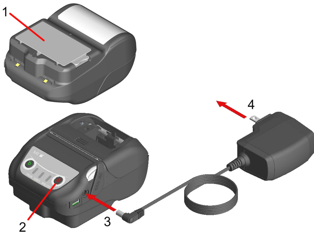
Abbildung 16-1 Aufladen im eingeschalteten Lademodus mit dem Netzteil
