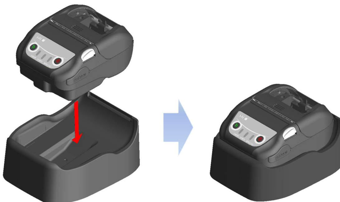
Abbildung 17-3 Drucker und Docking-Station-Verbindung
