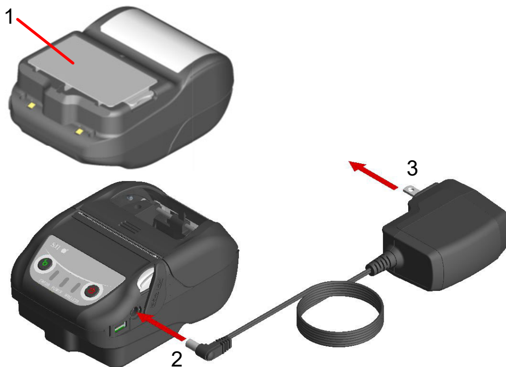
Abbildung 16-2 Aufladen im ausgeschalteten Lademodus mit dem Netzteil
