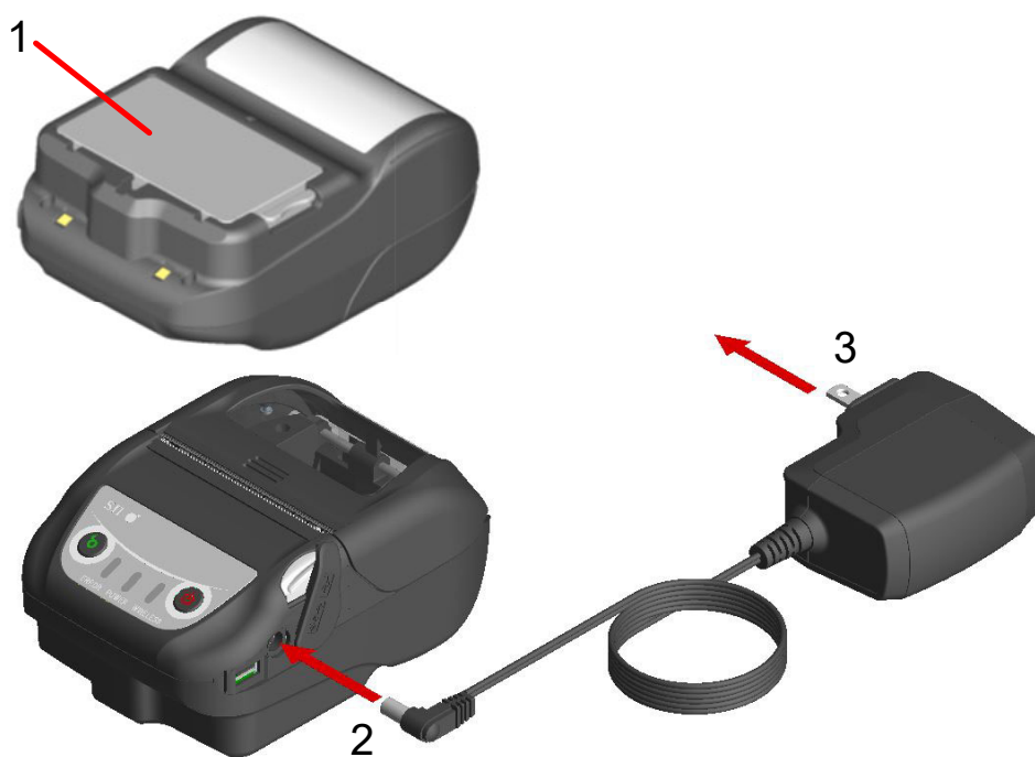
Illustration 16-2 Chargement en mode de chargement hors tension avec l'adaptateur c.a.
