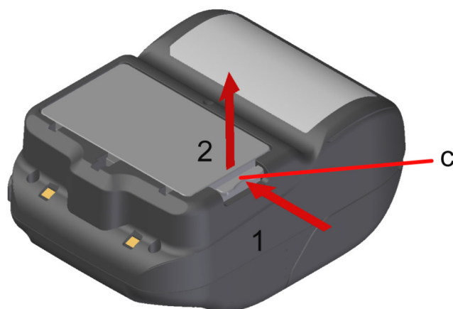
Illustration 8-1 Retrait de la batterie
