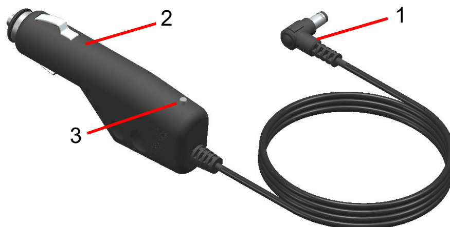
Illustration 18-1 Composants du chargeur de voiture (CC-A12-A1)
