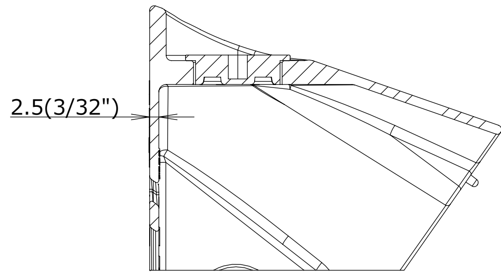
Sec A-A
